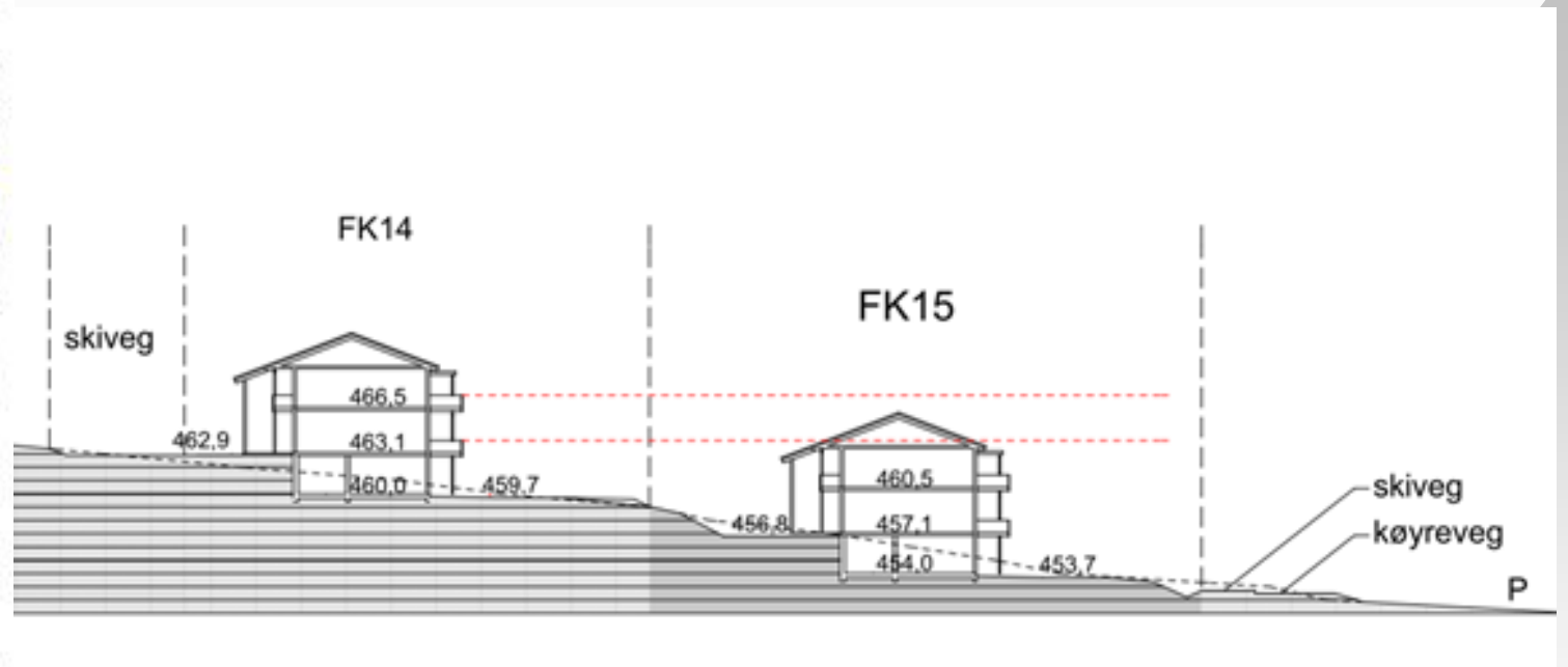
Snitt S1 gjennom FK14 og FK15
